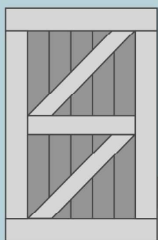
Double Z-brace (BD005)
